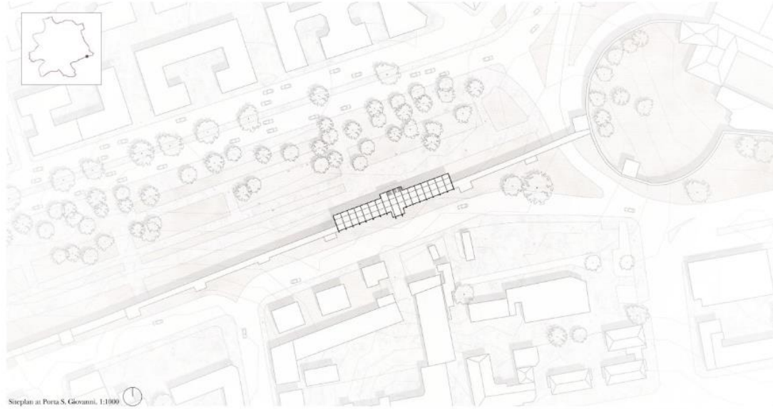
Siteplan at Porta S. Giovanni, 1:1000
